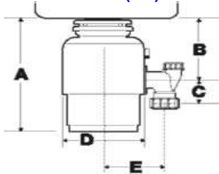
WYMIARY (mm)
