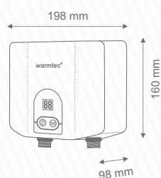
Wymiary
