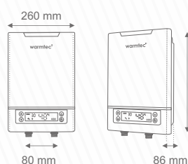
OPTISHOWER 7,5 kW
